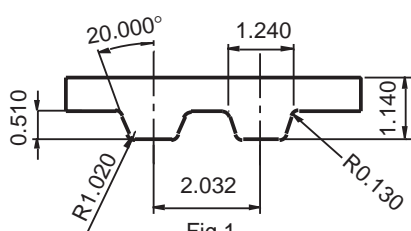
Fig.1 Passo 2.032mm (MXL)
