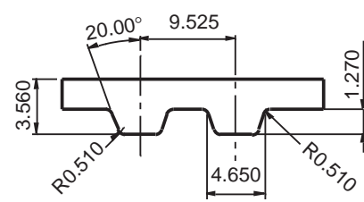
Fig.3 Passo 9.525mm (L)
