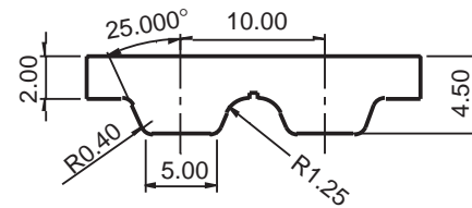
Fig.12 Passo 10.00mm (AT)
