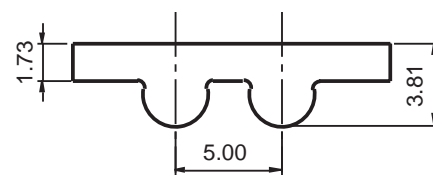
Fig.6 Passo 5.00mm (HTD)
